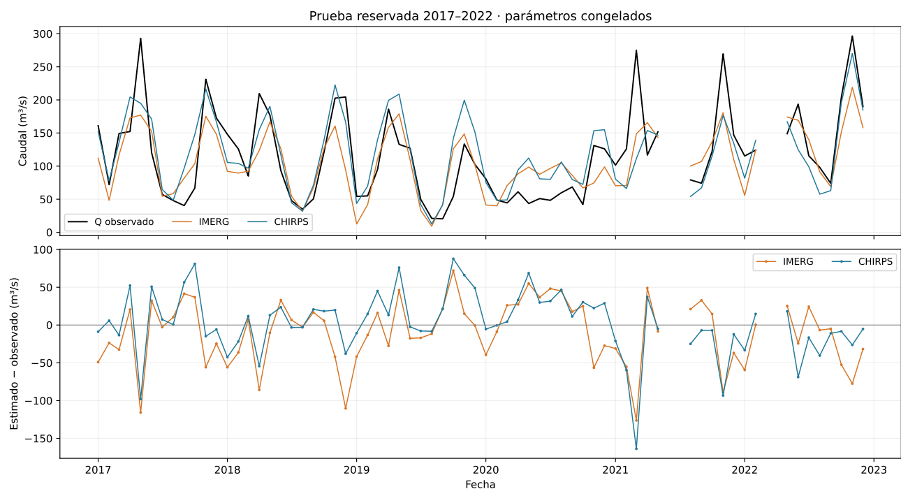
Figura 31: Series y errores de los modelos congelados, 2017–2022.
