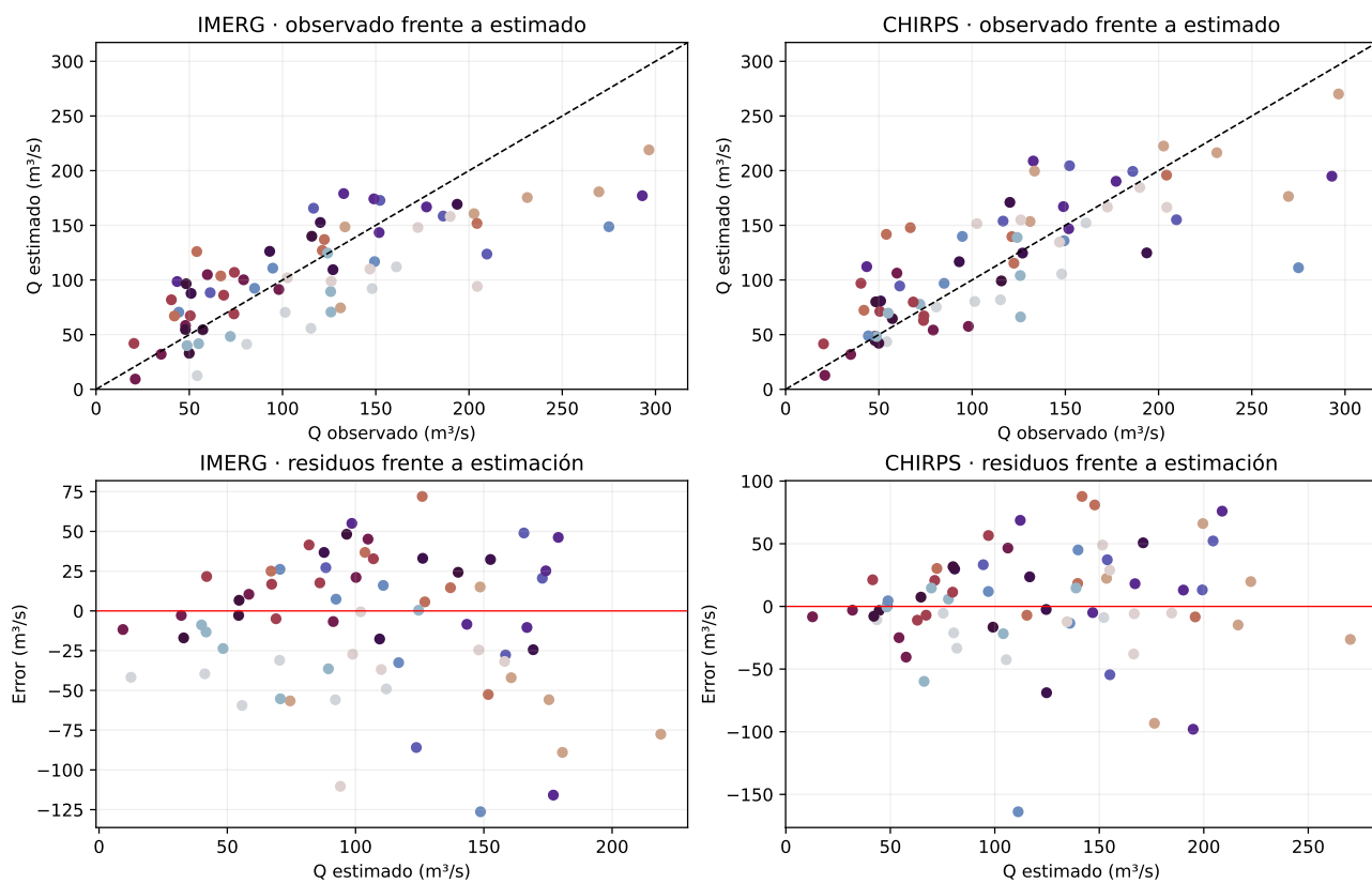
Figura 32: Predicciones y residuos frente al valor estimado.
